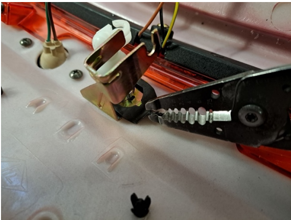
Ota penkin lukon kiinnitys lipsu pois.
