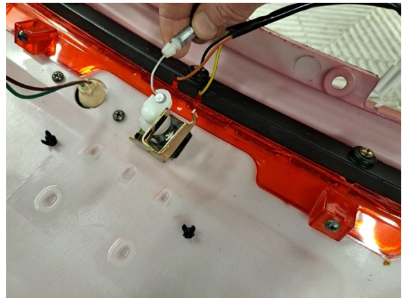
Ota penkin lukon vaijeri pois.
