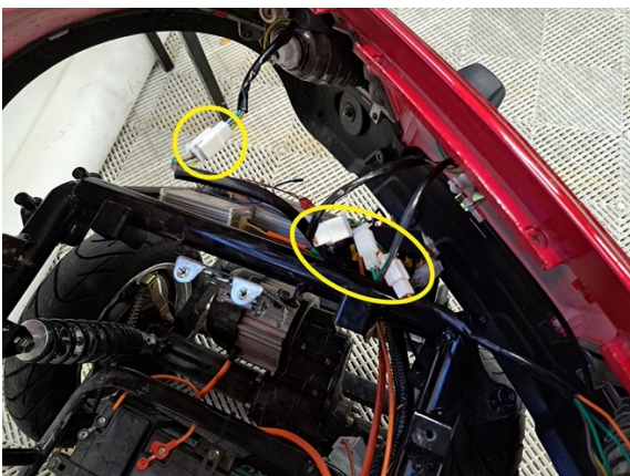
Nosta takakatetta ja avaa takavalojen liittimet.
