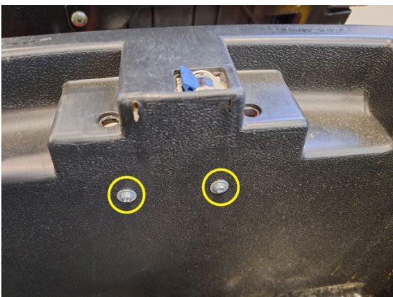
Irrota päävirtakytkimen kiinnitysruuvit. (ristipäämeisseli ph2).
