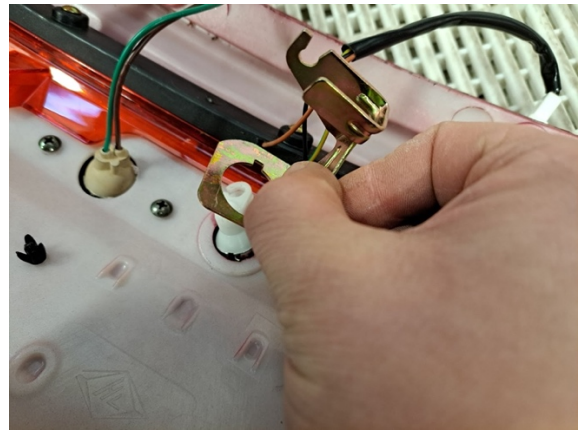
Ota penkin lukon vaijerin kiinnitys hässäkkä pois.
