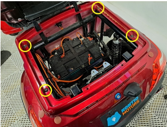
Irrota takakatteen kiinnityspultit. (hylsy 8 mm).
